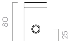
K200 SIDE K200 HP pulser BOTTOM
