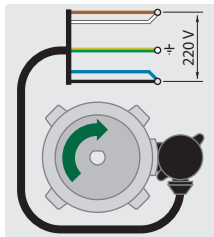
right rotation
