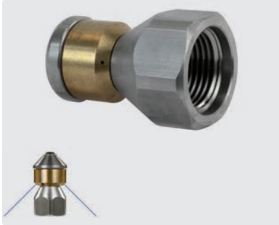
3/8" F. ⌀ 24 mm. Max. 250 bar
