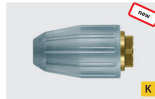
TR 20 F. Spray angle 20°. Max. 300 bar / 100 °C
